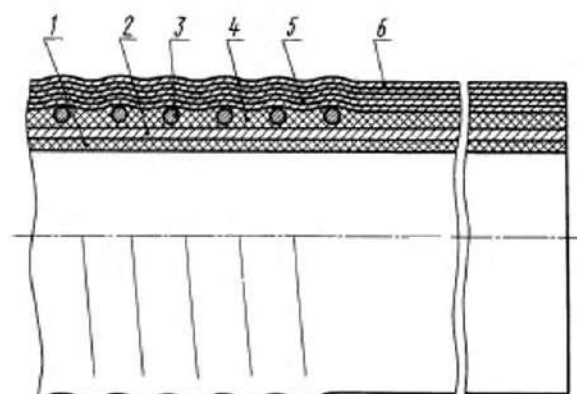
Схема конструкции рукава
